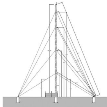
Ilustración 3 "Torre Riendada"
