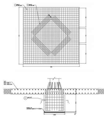
Ilustración 5 "Cimentación Tipo Losa"
