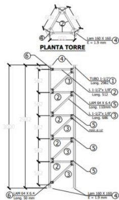
Ilustración 2 "Tramo tipo de 3m para torre riendada"
