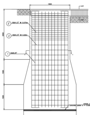
Ilustración 4 "Cimentación Tipo Caisson"
