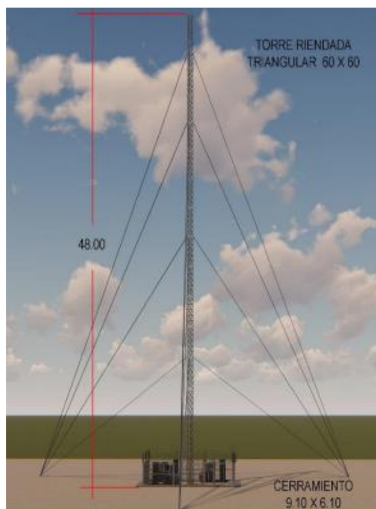
Ilustración 1 "Esquema de torre riendada"
