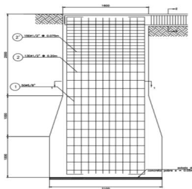
Ilustración 4 "Cimentación Tipo Caisson"
