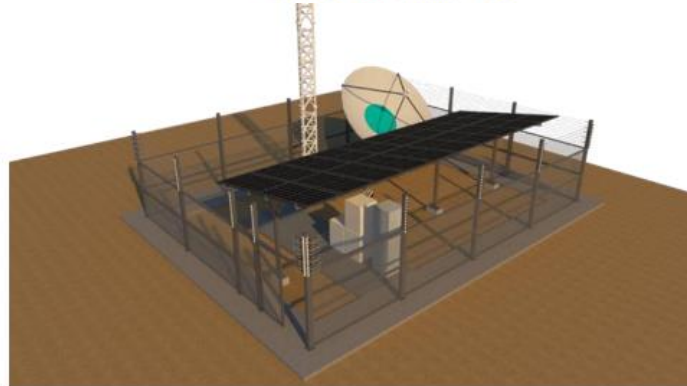
Ilustración 8 "Cerramiento en Malla"
