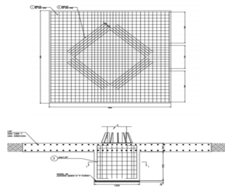
Ilustración 5 "Cimentación Tipo Losa"
