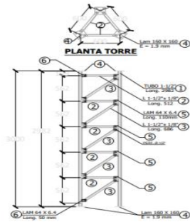
Ilustración 2 "Tramo tipo de 3m para torre riendada"
