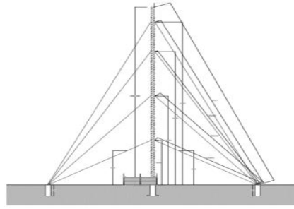
Ilustración 3 "Torre Riendada"
