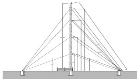
Ilustración 3 "Torre Riendada"
