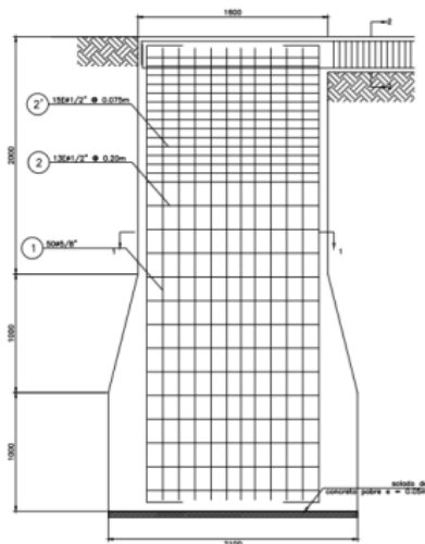
Ilustración 4 "Cimentación Tipo Caisson"
