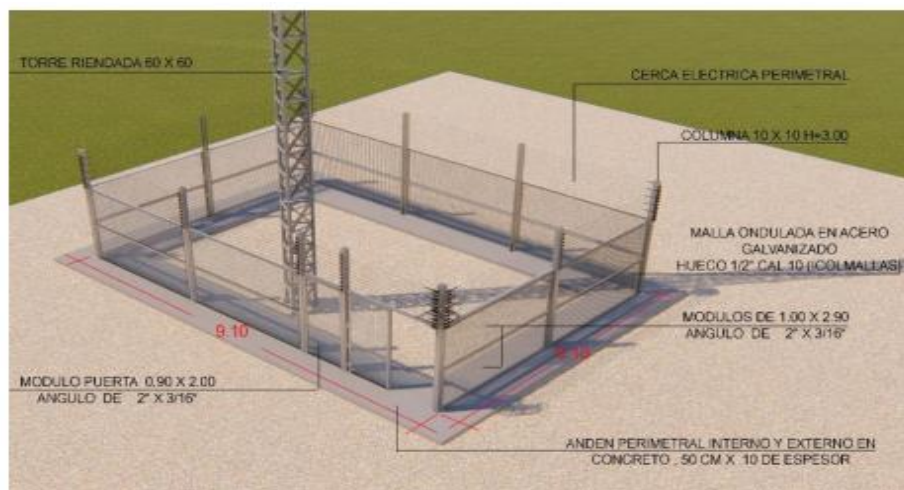
"Cerramiento en Malla"
