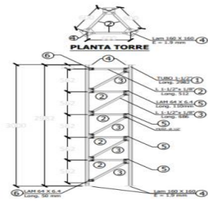
Ilustración 2 "Tramo tipo de 3m para torre riendada"
