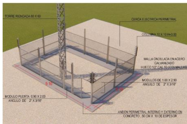
"Cerramiento en Malla"
