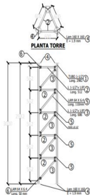
Ilustración 2 "Tramo tipo de 3m para torre rendada"
