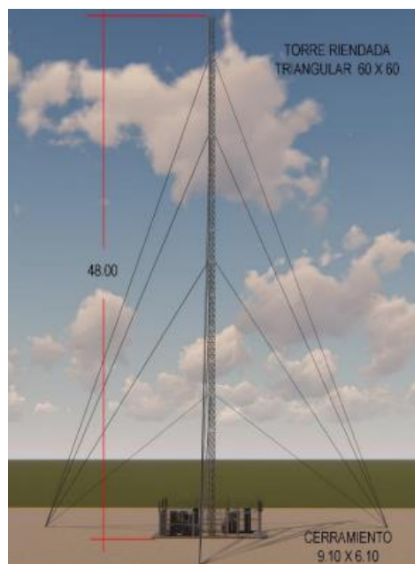
Ilustración 1 "Esquema de torre riendada"
