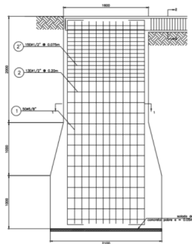
Ilustración 4 "Cimentación Tipo Caisson"
