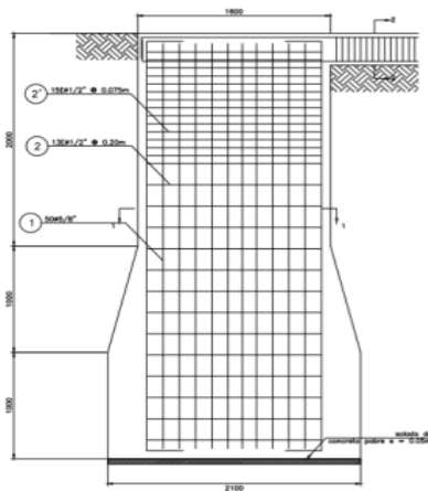
Ilustración 4 "Cimentación Tipo Caisson"
