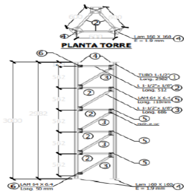
Ilustración 2 "Tramo tipo de 3m para torre riendada"
