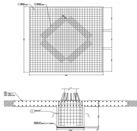
Ilustración 5 "Cimentación Tipo Losa"
