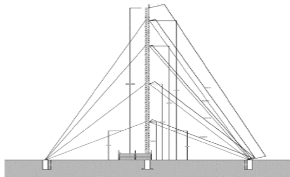
Ilustración 3 "Torre Riendada"
