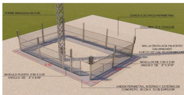
"Cerramiento en Malla"
