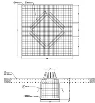
Ilustración 5 "Cimentación Tipo Losa"
