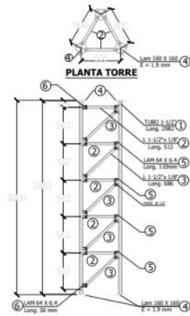
Ilustración 2 "Tramo tipo de 3m para torre riendada"
