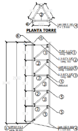
Ilustración 2ª Tramo tipo de 3m para torre riendada"
