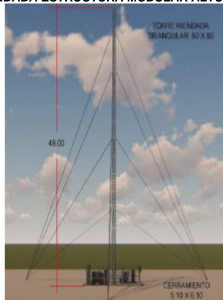
Ilustración 1 "Esquema de torre riendada"
