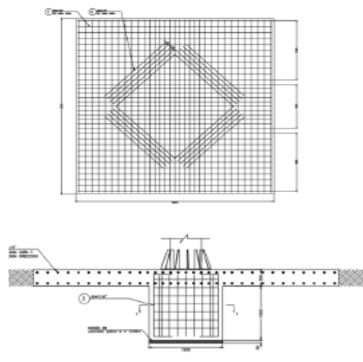
Ilustración 5ª Cimentación Tipo Losa"
