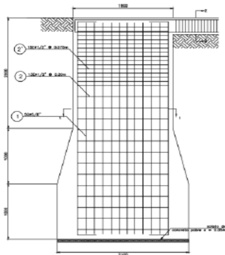
Ilustración 4ª Cimentación Tipo Caisson"
