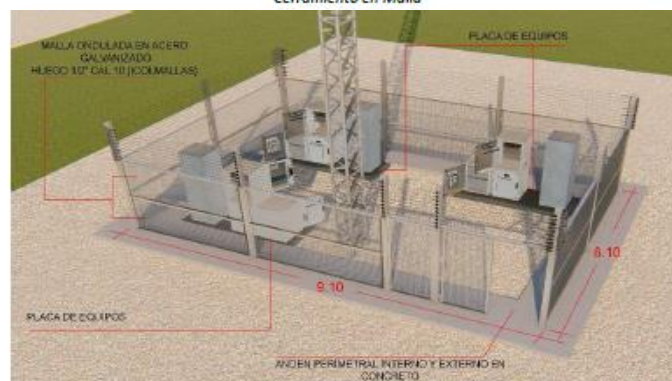
Ilustración 7 "Cerramiento en Malla"
