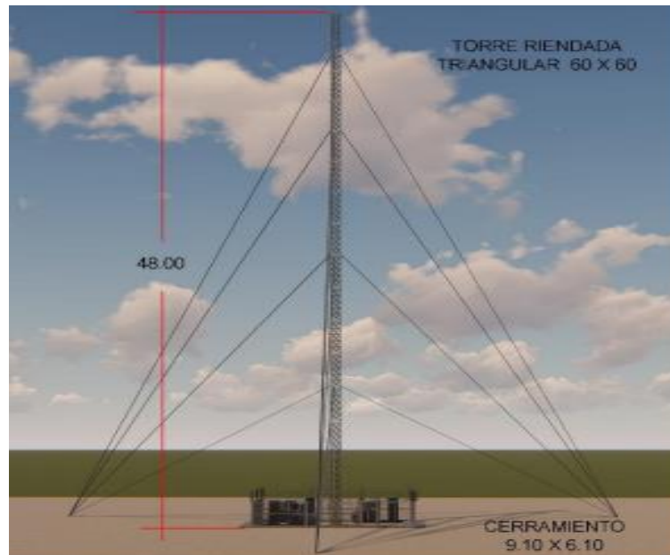
Ilustración 1 "Esquema de torre riendada"
