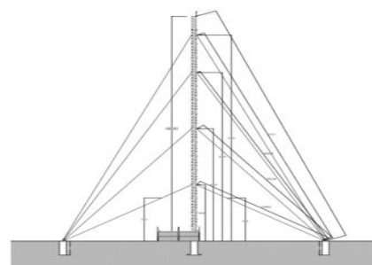
Ilustración 3 "Torre Riendada"
