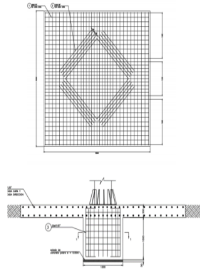
Ilustración 5 "Cimentación Tipo Losa"
