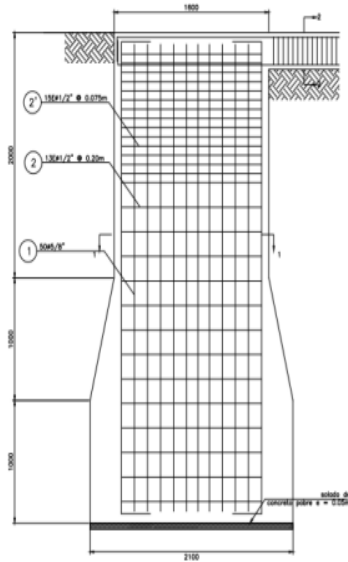
Ilustración 4 "Cimentación Tipo Caisson"
