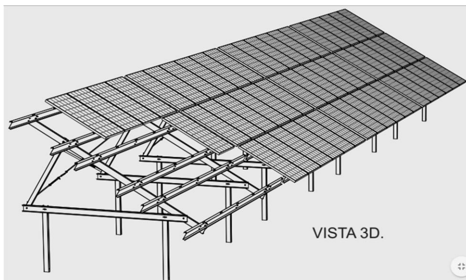
Figura 1 Vista 3D de la estructura metálica seleccionada
